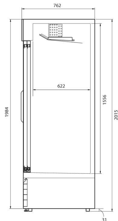
ВИД СБОКУ
