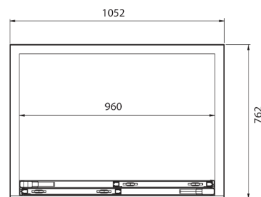
ВИД СВЕРХУ
