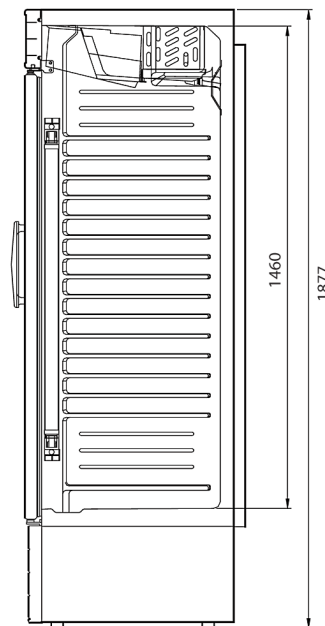
ВИД СБОКУ
