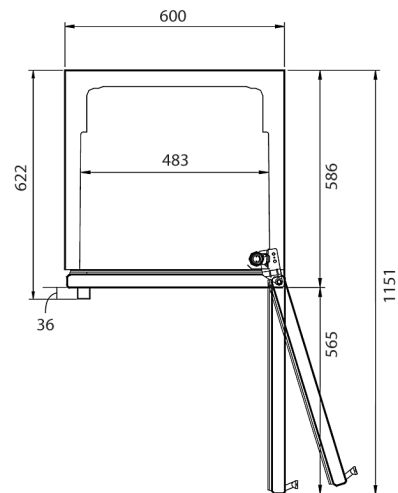
ВИД СВЕРХУ
